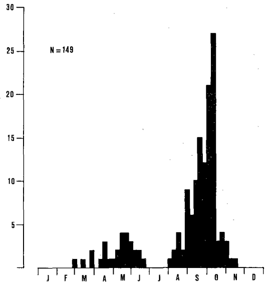
Figuur 7. Seizoenspatroon van Kleine Vliegenvanger, 1960—'79. Seasonal pattern of Red-breasted Flycatcher Ficedula parva in the Netherlands, 1960—'79
